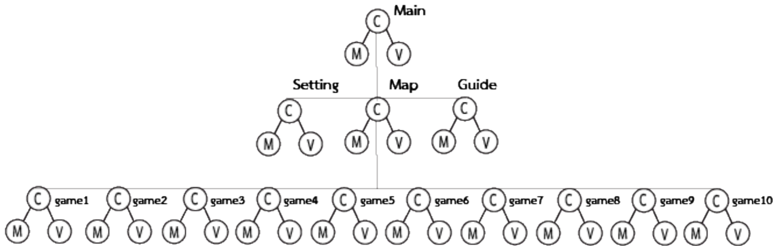
Figure 2.12 สถาปัตยกรรมแบบหลาย MVC
